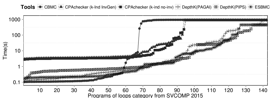
Figura 4.10: Tempo de verificação da categoria loops .
