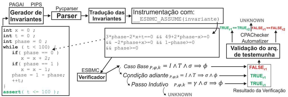
Figura 1.5: Passos da verificação executada através do DepthK .
