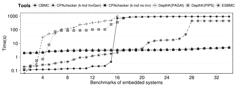
Figura 4.11: Tempo de verificação da categoria de sistemas embarcados.
